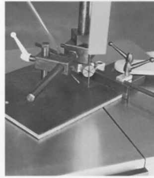
Dispositivo para cortes circulares Circular cutting guide
