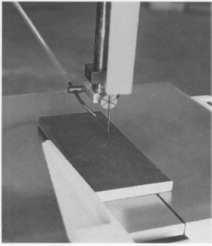
Regla cortes paralelos Parallel guide rule
